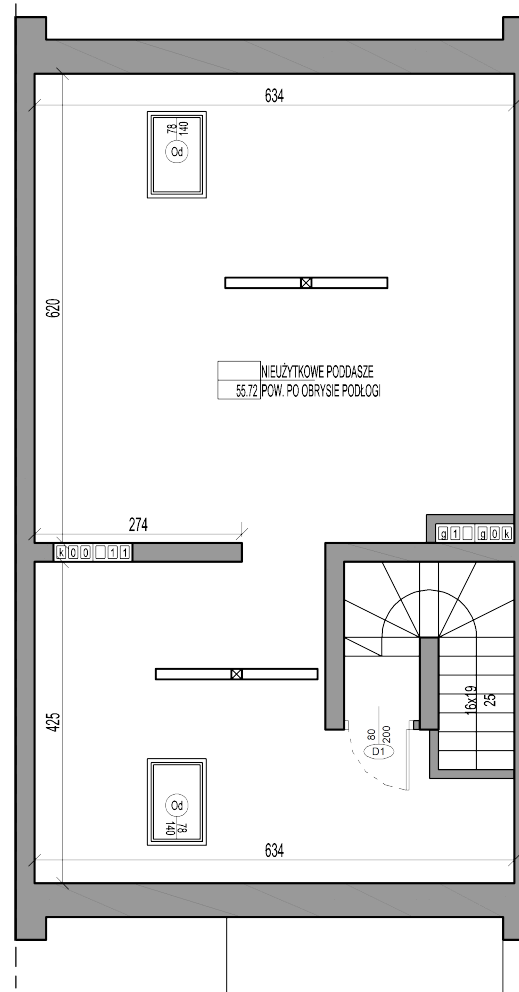
RZUT PODDASZA NIEUŻYTKOW. LOKAL 2
