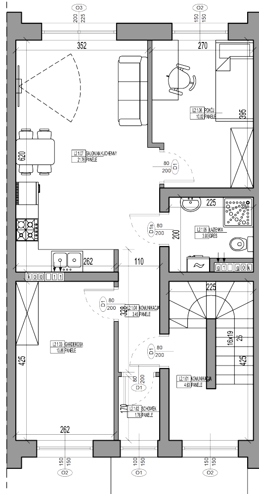
RZUT PIĘTRA LOKAL 2
